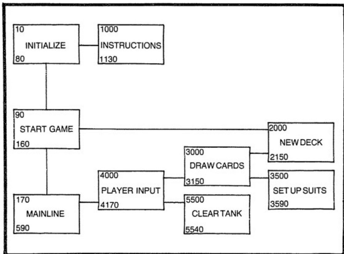
Fig. L-1. Program template for Lapidis.
