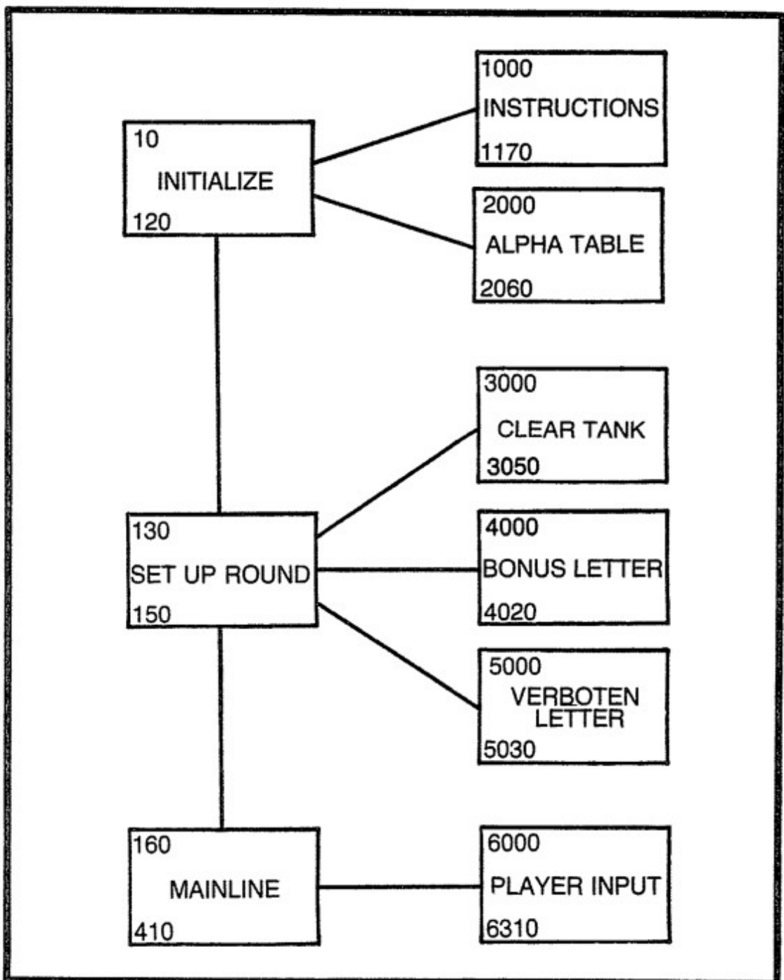
Fig. V-1. Program template for Verboten.
