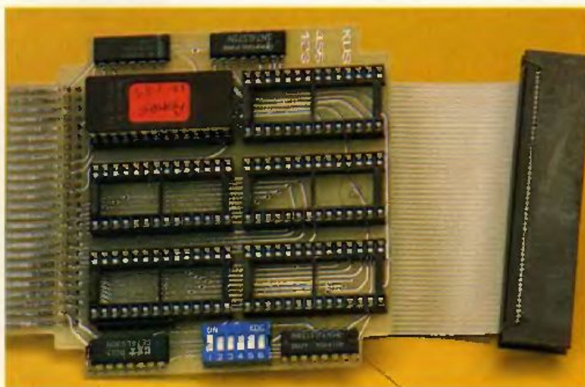
Diferentes conexiones para las ROM's en el interior del interface. En la parte inferior de la placa se pueden observar los switches para seleccionar cada una de las pastillas ROM.
